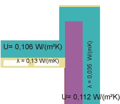
Attikaausbildung Altbau
