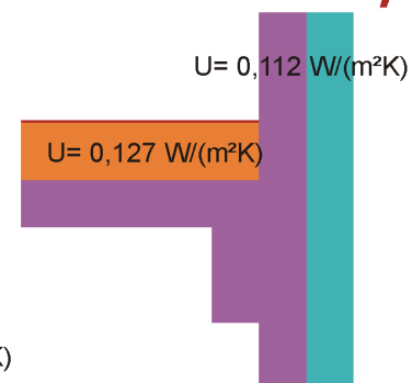
Verbindung Schwimmhalle- Schalthele Altbau
